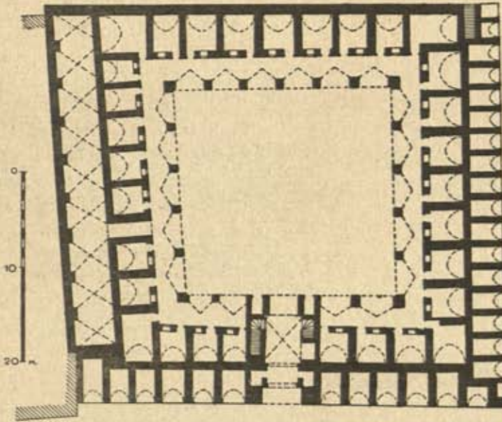
FIG. 19. — ALEP. Le khan des Chaudronniers (milieu du XVI e siècle) : plan du rez-de-chaussée. Des boutiques faisant partie du souk sur lequel ouvre la porte du khan sont placées au nord (à droite) et à l'est (en bas). Les magasins des négociants s'ouvrent sur une galerie voûtée qui fait tout le tour de la cour; une longue écurie règne tout le long de la façade sud. L'étage (où sont les logements) reproduit grosso modo la même disposition.
