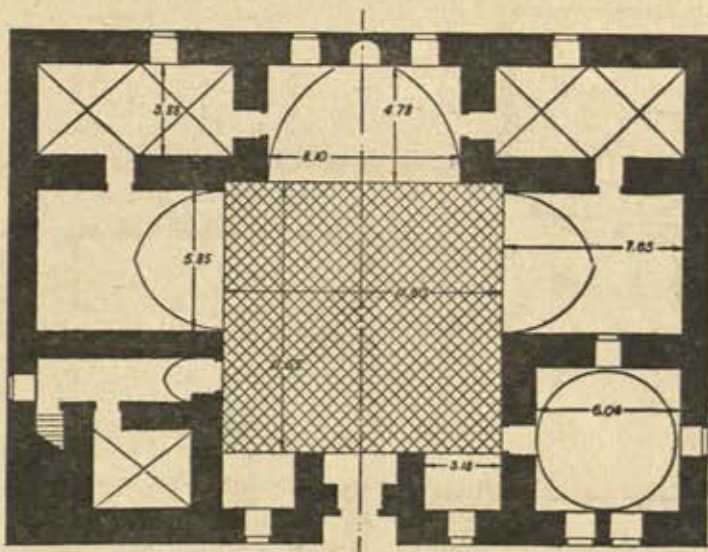
FIG. 961r. — DAMAS, Madrasa Sâhibiya (entre 1233 et 1245). — Mausolée à coupole, salle de prière, deux iwâns et deux salles voûtées, latrines.
