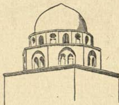
FIG. 3. — DAMAS. Coupole (fin du XII e siècle). — Deux zones polygonales créent une heureuse transition entre le cube de base et la sphère de la coupole.
